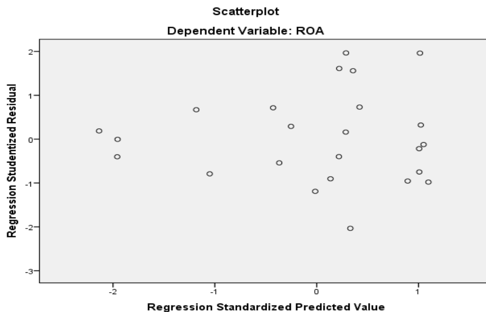
Gambar 4.1 Uji Heteroskedastisitas
